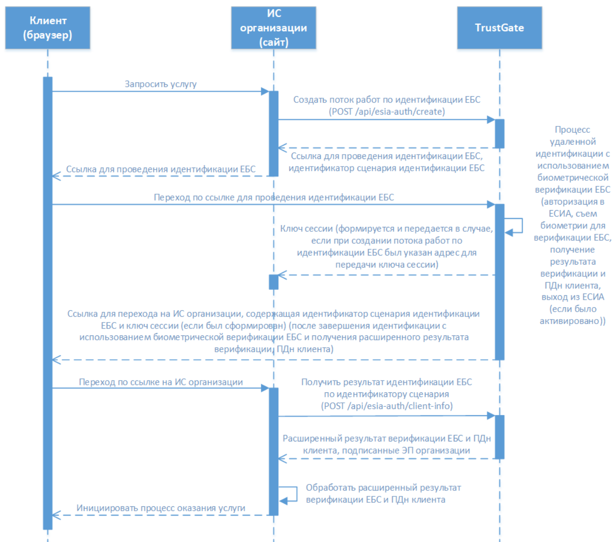
Рисунок 1 – Схема работы для удаленной идентификации клиентов с использованием биометрической верификации в ЕБС при непосредственном взаимодействии клиента (браузера) с системой TrustGate.
