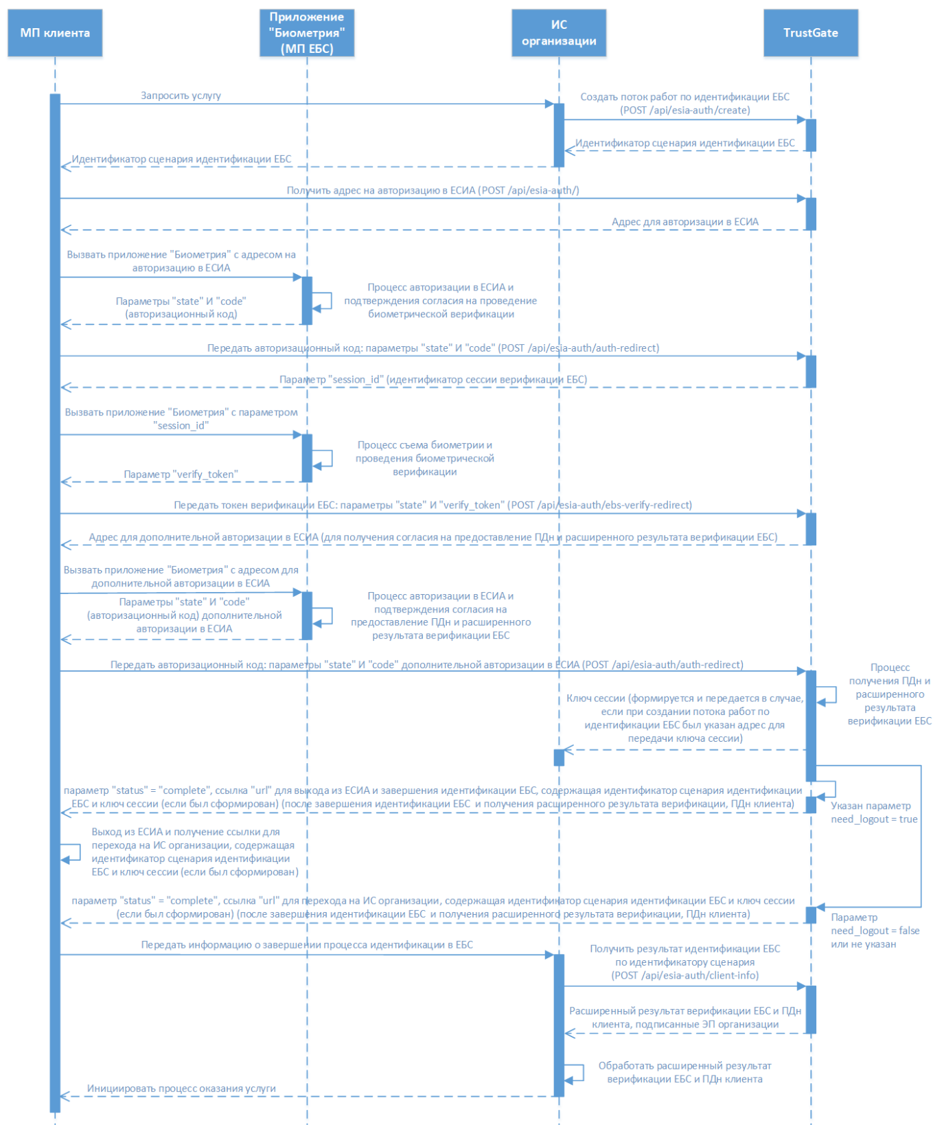
Рисунок 3 - Схема работы для удаленной идентификации клиентов с использованием биометрической верификации в ЕБС через мобильное приложение.
