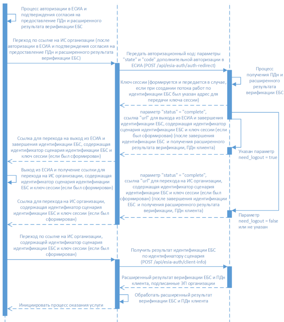
Рисунок 2 - Схема работы для удаленной идентификации клиентов с использованием биометрической верификации в ЕБС при непосредственном взаимодействии клиента (браузера) только с ИС КО (продолжение).
