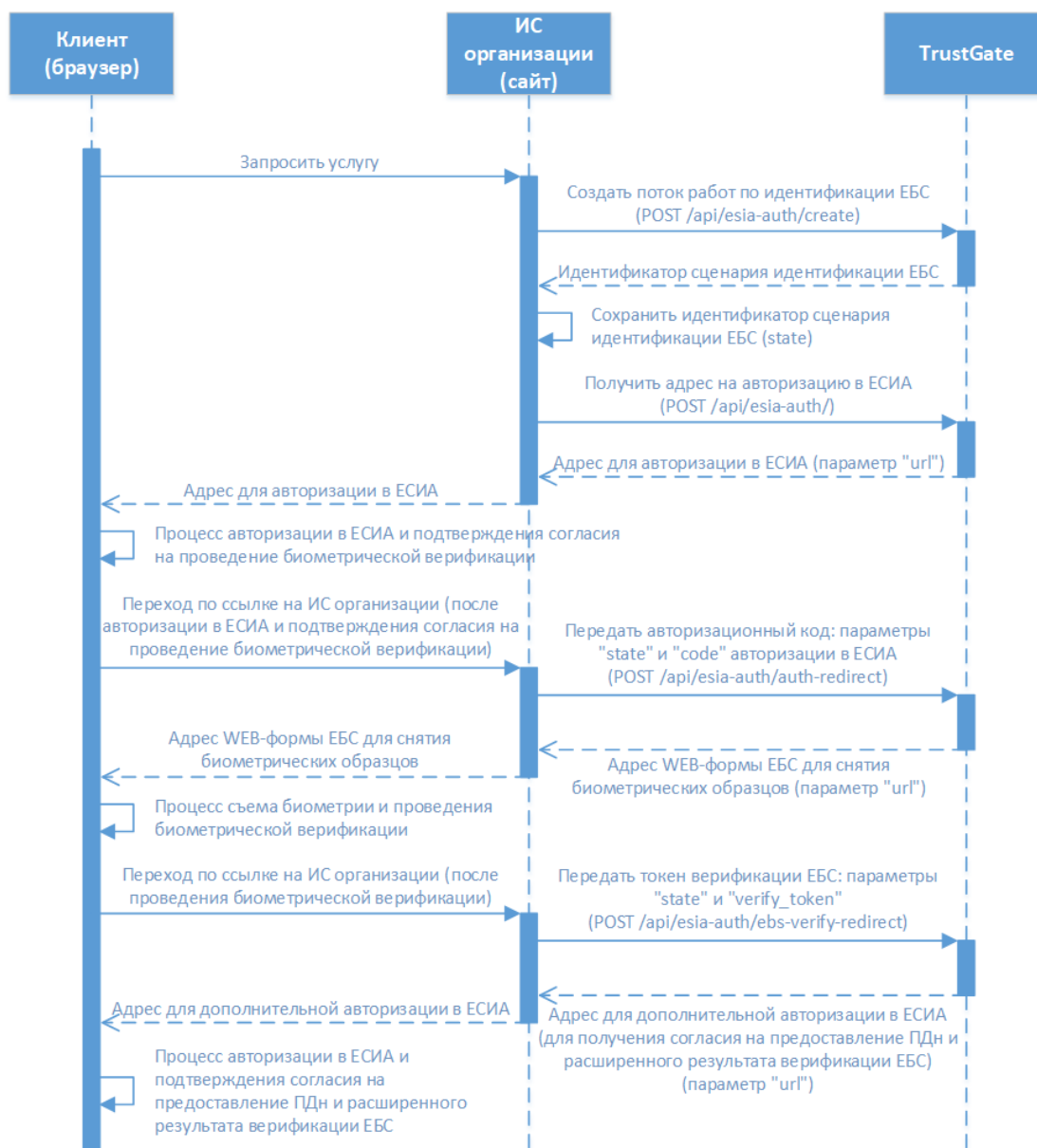
Рисунок 2 - Схема работы для удаленной идентификации клиентов с использованием биометрической верификации в ЕБС при непосредственном взаимодействии клиента (браузера) только с ИС КО (начало).
